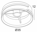
VISOR 39 24144 0030
