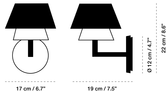
GALA MINI Pantalla doble Double shade
